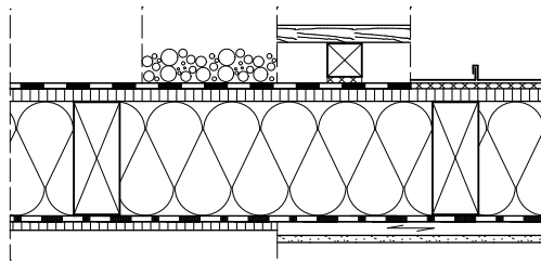
Abb. 2.4 Nicht belüftetes Flachdach mit Vollwärmung in der Tragkonstruktion (ggf. mit Installationsebene)
